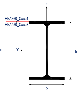
Fig. 5.17.3 Steel columns
